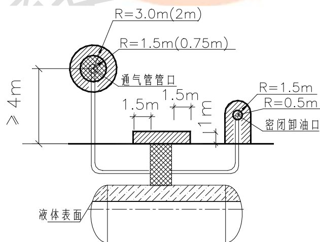
图 1 埋地卧式汽油储罐爆炸危险区域划分
