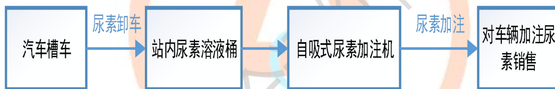
图 2-5 尿素加注站工艺流程简图
